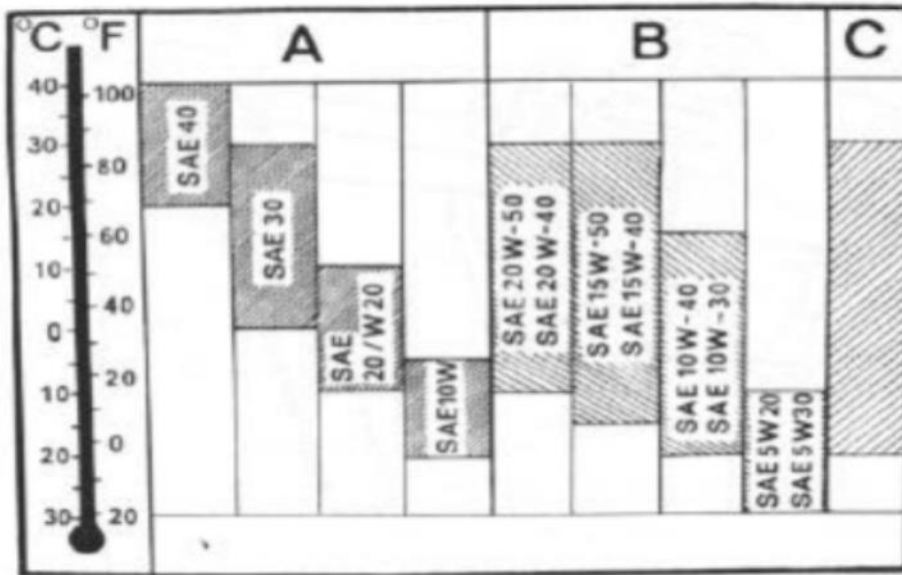
Bild M 43. Motoröl-Viskositätsklassen
